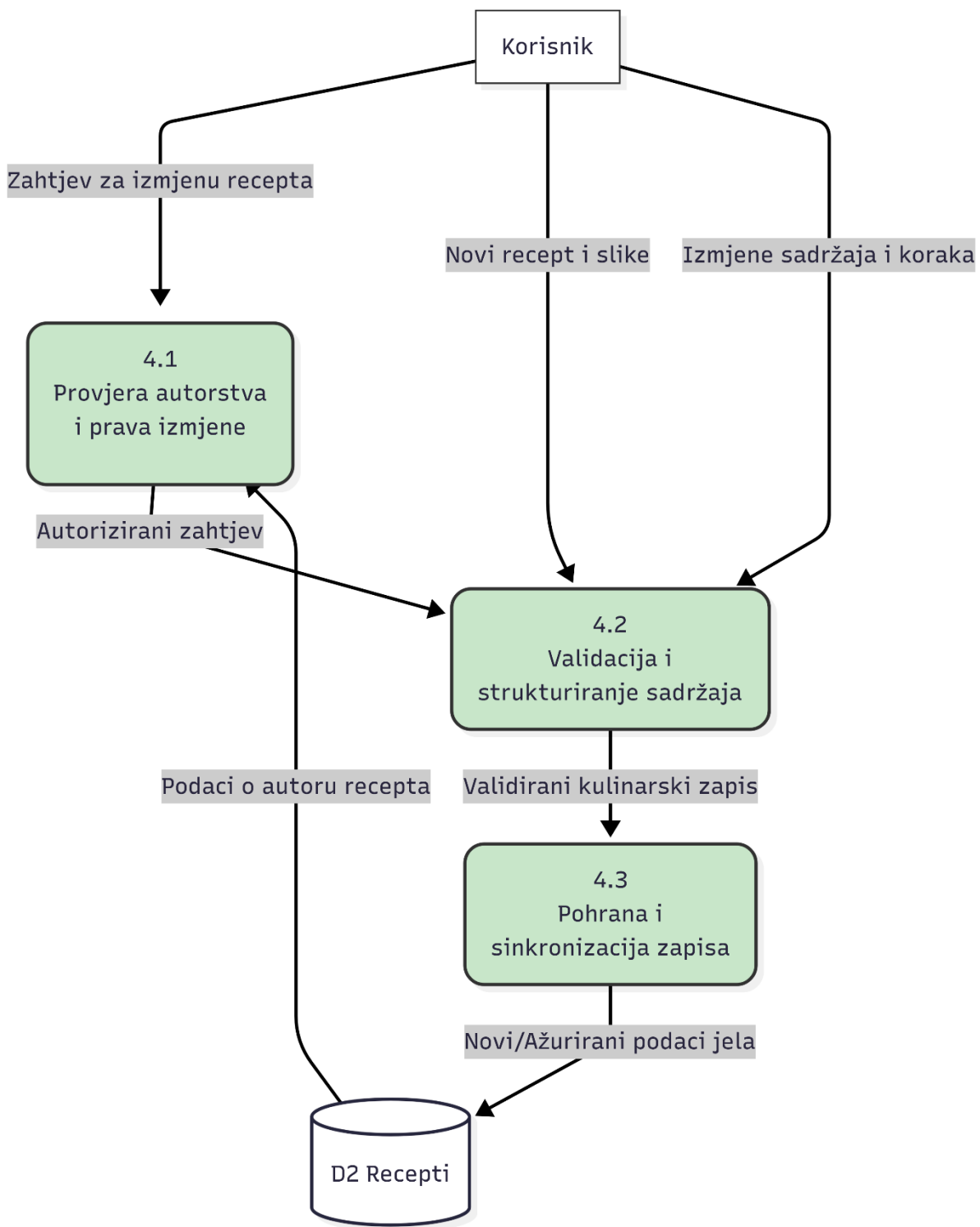
Slika 4.3 Dijagram razine 2
