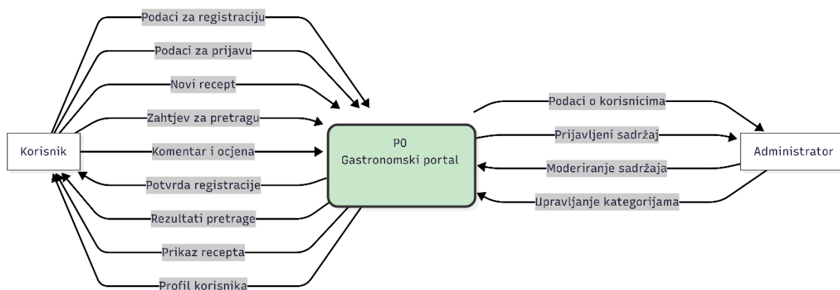
Slika 4.1 Dijagram razine 0
